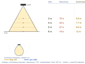
Ausleuchtung (Richtwert) 1110QP - 1110 (QP) 36W 4000K Halbwinkel 44° (typ.) (C0) 40° (typ.) (C0)
