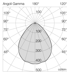
Ausleuchtung (Richtwert) 1110QP - 1110 (QP) 36W 4000K Halbwinkel 44° (typ.) (C0) 40° (typ.) (C0)
