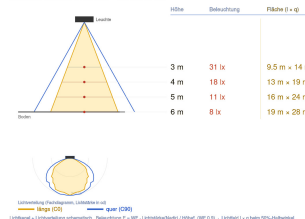
Ausleuchtung (Richtwert) 2156LC4100D1 - 100W 4000K 1000lm Halbwertske (HP) 180° (30°) 45° 60° 75° 90° 105° 120°
