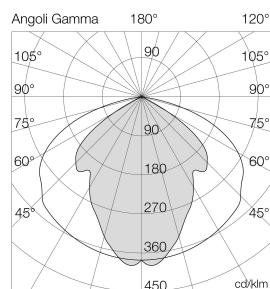
Ausleuchtung (Richtwert) 2156LC4100D1 - 100W 4000K 1000lm Halbwertske (HP) 180° (30°) 45° 60° 75° 90° 105° 120°
