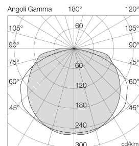
Ausleuchtung (Richtwert) 2156LT - HAN 2156LT3120 - 17281 lm Halbwinkel (50°) 105° 120° 180°
