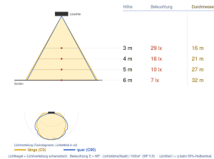
Ausleuchtung (Richtwert) 2156LT - HAN 2156LT3120 - 17281 lm Halbwinkel (50°) 105° 120° 180°
