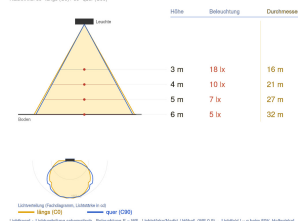
Ausleuchtung (Richtwert) 2156LT - HAN 2156LT5070 - 11048 lm Halbwinkel (50°) (50°) (50°) (50°)
