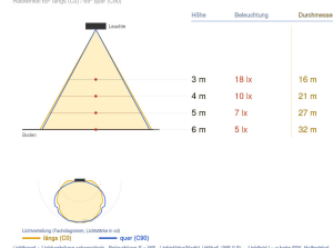
Ausleuchtung (Richtwert) 2156LT - HAN 2156LT5070 - 11048 lm Ausleuchtung (Richtwert) (lx) (Richtwert) (lx)
