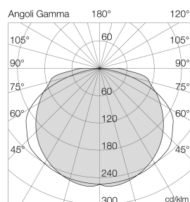
Ausleuchtung (Richtwert) 2156LT - HAN 2156LT5070 - 11048 lm Halbwinkel 50° (typ.) 50° (typ.) 50° (typ.)
