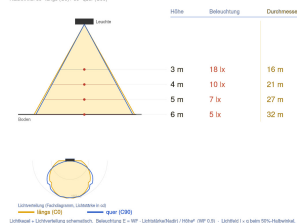
Ausleuchtung (Richtwert) 2156LT - HAN 2156LT5070 - 11048 lm Halbwinkel 50° (typ.) 50° (typ.) 50° (typ.)
