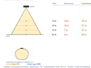
Ausleuchtung (Richtwert) 2156LT - HAN 2156LT9080 - 11000 lm Halbwinkel 22° (typ.) 22° (typ.) 22°
