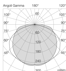
Ausleuchtung (Richtwert) 2156LT - HAN 2156LT9080 - 11000 lm Halbwinkel 120° (CRI 90, 4000K, 80W)
