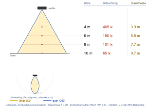
Ausleuchtung (Richtwert) 3001W44 - 1400 3001W44070 (1700 lx) Halbwinkel 20° (Ang. 105°) 20° (Ang. 105°)
