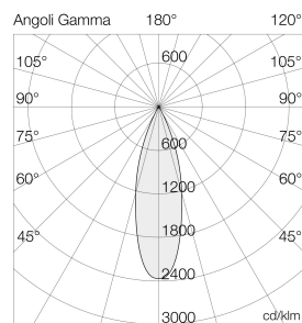
Ausleuchtung (Richtwert) 3001W44 - 1400 3001W44070 (1700 lx) Halbwinkel 20° (Ang. 105°) 20° (Ang. 105°)
