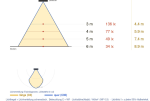
Ausleuchtung (Richtwert)
