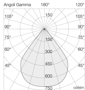
Ausleuchtung (Richtwert) 600318 - 18x18 6003DOGE (18) 40W 4000K Halbwinkel 27° (Ang. 0.5) 27° (Ang. 0.5)
