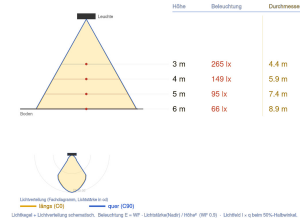
Ausleuchtung (Richtwert) 600318 - 18x18 6003DOGE (18) 40W 4000K Halbwinkel 27° (Ang. 0.5) 27° (Ang. 0.5)
