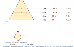
Ausleuchtung (Richtwert)
