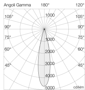
Ausleuchtung (Richtwert) 6104C1 - 1080 x 1080 (2017) - 12000 lm Halbwinkel 11° (Ang. CIE) - 8° (ang. CIE)
