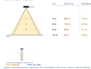
Ausleuchtung (Richtwert) 6104C1 - 1080 x 1080 (2017) - 12000 lm Halbwinkel 11° (Ang. CIE) - 8° (ang. CIE)
