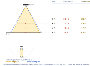
Ausleuchtung (Richtwert) 6200Q1 - 18W/3000K/180° - 1700 lm Halbwinkel 10° (Ang. 0.5) / 17° (Ang. 0.25)
