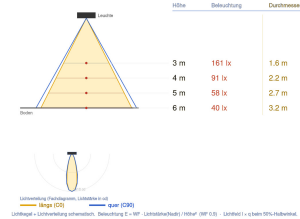
Ausleuchtung (Richtwert) 6200Q1 - 1400mm x 1400mm - 10000 lm Halbwinkel 10° (Ang. 0.5) / 10° (Ang. 0.5)
