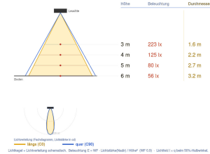
Ausleuchtung (Richtwert) 6200Q1 - 1400mm x 1400mm - 12W Halbwinkel 10° (Ang. 0.5) / 17° (Ang. 0.9)
