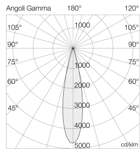
Ausleuchtung (Richtwert) 6200Q1 - 1400mm x 1400mm - 12W Halbwinkel 10° (Ang. 0.5) / 17° (Ang. 0.9)
