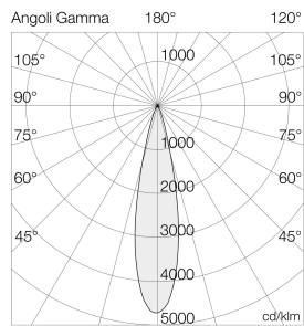
Ausleuchtung (Richtwert) 6200Q1 - 18W/4000K/4000K - 1800lm Halbwinkel 10° (Ang. 0.5) / 17° (Ang. 0.25)
