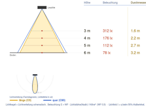
Ausleuchtung (Richtwert) 6200Q1 - 18W/4000K/4000K - 1800lm Halbwinkel 10° (Ang. 0.5) / 17° (Ang. 0.25)
