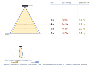
Ausleuchtung (Richtwert) 6200Q1 - 140x140mm (Q1) - 26W 4000K Halbwinkel 10° (Ang. 0.5) / 17° (Ang. 0.9)
