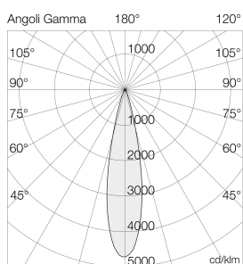
Ausleuchtung (Richtwert) 6200Q1 - 140x140mm (Q1) - 26W 4000K Halbwinkel 10° (Ang. 0.5) / 17° (Ang. 0.9)
