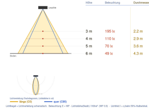
Ausleuchtung (Richtwert) 6200Q33012SD - 1440 lm (3000K) - 12W Halbwinkel 20° (typ.) / 10° (opt.)
