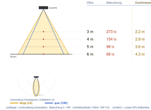
Ausleuchtung (Richtwert) 6200Q33018CD - 18W 3000K (Q3) - 12000 lm Halbwinkel 30° (Q3) / 10° (Q3)
