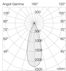
Ausleuchtung (Richtwert) 6200Q33018CD - 18W 3000K (Q3) - 12000 lm Halbwinkel 30° (Q3) / 10° (Q3)
