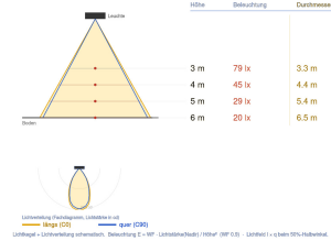
Ausleuchtung (Richtwert) 6200Q63008CL - 8W 3000K CLEO (Q6) 8W 3000K Halbwinkel 20° (typisch) 20° (typisch)
