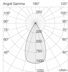
Ausleuchtung (Richtwert) 6200Q63008CL - 8W 3000K CLEO (Q6) 8W 3000K Halbwinkel 20° (typisch) 20° (typisch)
