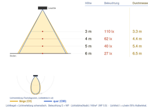
Ausleuchtung (Richtwert) 6200Q63012CD - 12W 3000K CLEO (Q6) 12W 3000K Halbwinkel 20° (typisch) 20° (typisch)
