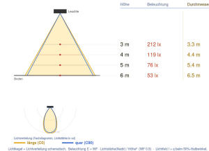
Ausleuchtung (Richtwert) 6200Q63026CD - 1x26W/3000K/2600lm Halbwinkel 20° (Ang. 0.5) 27° (Ang. 0.5)
