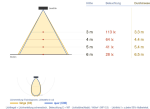
Ausleuchtung (Richtwert) 6200Q6 - 12W 4000K DALI - 1200 lm Halbwinkel 20° (typ.) 27° (max. 30°)
