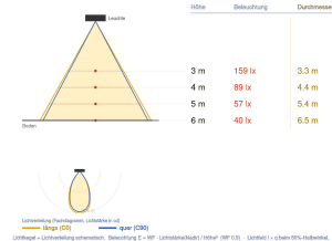
Ausleuchtung (Richtwert) 6200Q64018BD - 18W 4000K (Q6) - 12145 lm Halbwinkel 20° (Q6) - 20° (Q6) - 20° (Q6)
