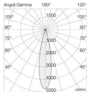
Ausleuchtung (Richtwert) 6200R1 - 12W 6200R13012 - 1 x LED 12W Halbwinkel 10° (Ang. 0.5) 10° (Ang. 0.5)
