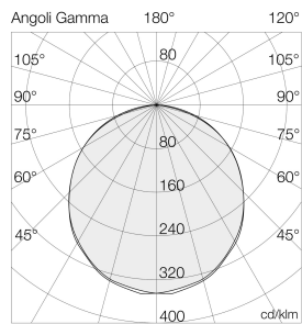
Ausleuchtung (Richtwert) 7012G33020ES - 1400 mm x 1400 mm x 1400 mm Haken mit 80° (G3) - 80° (G3)
