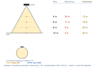
Ausleuchtung (Richtwert) 7012G33020ES - 1400 mm x 1400 mm x 1400 mm Haken mit 80° (G3) - 80° (G3)
