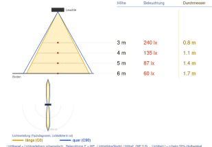
Ausleuchtung (Richtwert)
