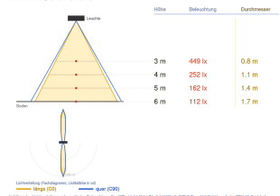
Ausleuchtung (Richtwert)
