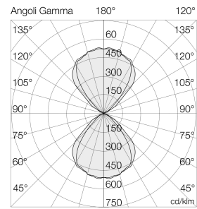
Ausleuchtung (Richtwert) 7022/88 - HAN 7022894014 | 1147 lm Halbwinkel 48° längs (D3) / 51° quer (D90)
