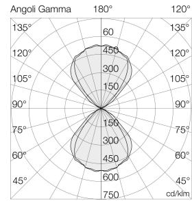
Ausleuchtung (Richtwert) 7022/88 - HAN 70228/4014 | 1147 lm Halbwinkel 48° längs (D3) / 51° quer (D90)
