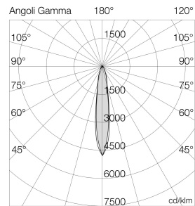
Ausleuchtung (Richtwert) 7022M1 - HAN 7022M14014 | 1269 lm Halbwinkel 6° (längs (D8) / 9° quer (D90))
