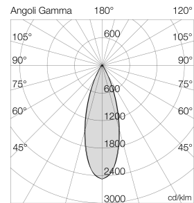
Ausleuchtung (Richtwert) 7022M3 - HAN 7022M34014 | 1208 lm Halbwinkel: 17° längs (CG) / 17° quer (CG)
