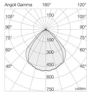
Ausleuchtung (Richtwert) 7022MB - HAN 7022MB4034 | 1107 lm Halbwinkel 49° längs (C0) / 51° quer (C90)
