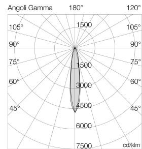
Ausleuchtung (Richtwert) 7022/51 - HAN 7022/1-4095 | 300 lm Halbwinkel 15° längs (D3) / 14° quer (D90)
