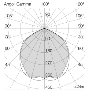
Ausleuchtung (Richtwert) 7025IPR - HAN 7025PR0000 | 3000 lm Halbwinkel 56° längs (D3) / 55° quer (D90)
