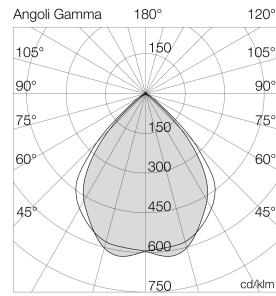
Ausleuchtung (Richtwert) 7031PR - 50W 3000K 50° - 1000lm Halbwinkel 50° (50° - 50° oder 200°)
