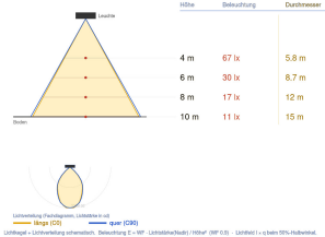
Ausleuchtung (Richtwert)
