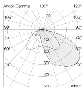
Ausleuchtung (Richtwert) 7036A54050GL (50W) 4000K Silber Halbwinkel 55° (30°/150° beam (30°))
