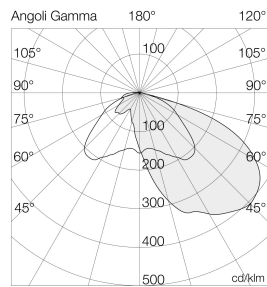
Ausleuchtung (Richtwert) 7038A53130GD - MAX 7038A53130GD - 130W 3000K Haben Sie 100° (100°) - 100° (100°)
