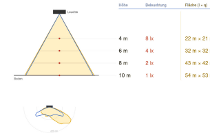
Ausleuchtung (Richtwert)
