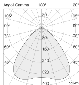
Ausleuchtung (Richtwert) Flutlichter 7038 IPADEL (S9) 50W 4000K Silber Halbwinkel 42° (S9) 40° (S9)
