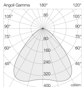
Ausleuchtung (Richtwert) Flutlichter 100W (S9) - 105W (S9) Halbkegel 42° (S9) - 42° (S9)
