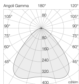
Ausleuchtung (Richtwert) Flutlichter 130W (S9) 4000K Silber Haben Sie 40° (S9) 4000K Silber (S9)
