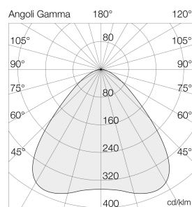
Ausleuchtung (Richtwert) Flutlichter 175W (S9) - 4000K (S9) Haben Sie 47 Strahler (S9) - 4000K (S9)
