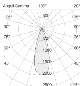
Ausleuchtung (Richtwert) 7039C34105GL - 105W 4000K Silber - 32°
