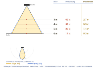
Ausleuchtung (Richtwert) 7050M6 - 5W 3000K (CRI > 90) Halbwinkel 24° (Ang. 250°) / 24° (Ang. 250°)
