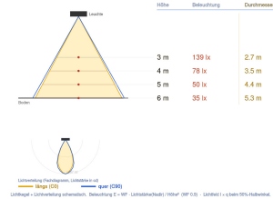
Ausleuchtung (Richtwert) 7050M63010BL - 10W/3000K/30° - 1780 lx Halbwinkel 34° (Ang. 33°) - 33° quer (33°)
