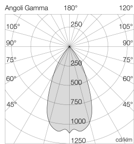
Ausleuchtung (Richtwert) 7050M63015SL - 15W/3000K/30° - 1170 lm Halbwinkel 24° (Ang. 23°) - 23° quer (23°)
