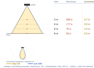
Ausleuchtung (Richtwert) 7050M63015SL - 15W/3000K/30° - 1170 lm Halbwinkel 24° (Ang. 23°) - 23° quer (23°)
