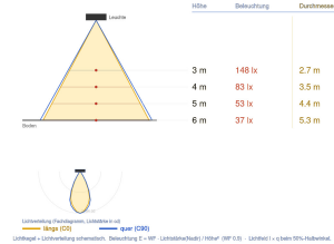
Ausleuchtung (Richtwert) 7050M64010SL - 10W 4000K (CRI > 90) Halbwinkel 24° (Ang. 105° / 24° quer 105°)
